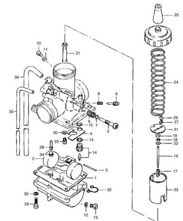
FIG.5 CARBURETOR
