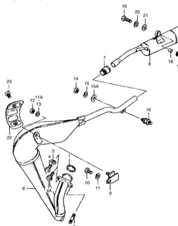
FIG.7 MUFFLER
