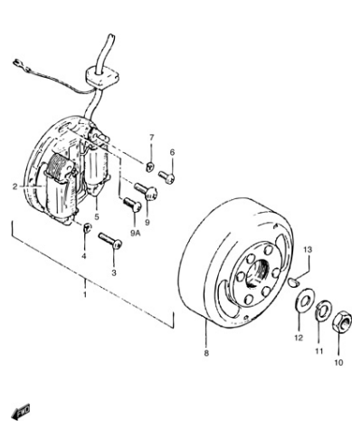
FIG.13 MAGNETO
